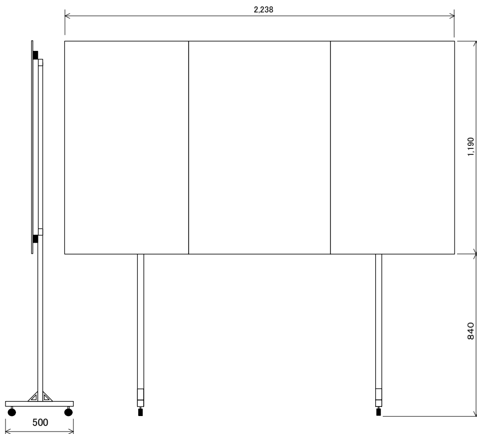
分割ボード外形図(前面)
